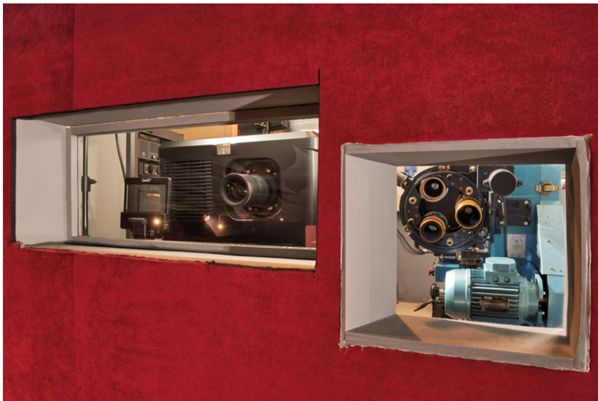
Salle 1 : fenêtres de projection. Projecteurs numérique Barco (à gauche) et argentique Cinemeccanica (à droite). 71, Autun, 3-5 rue Pernette
