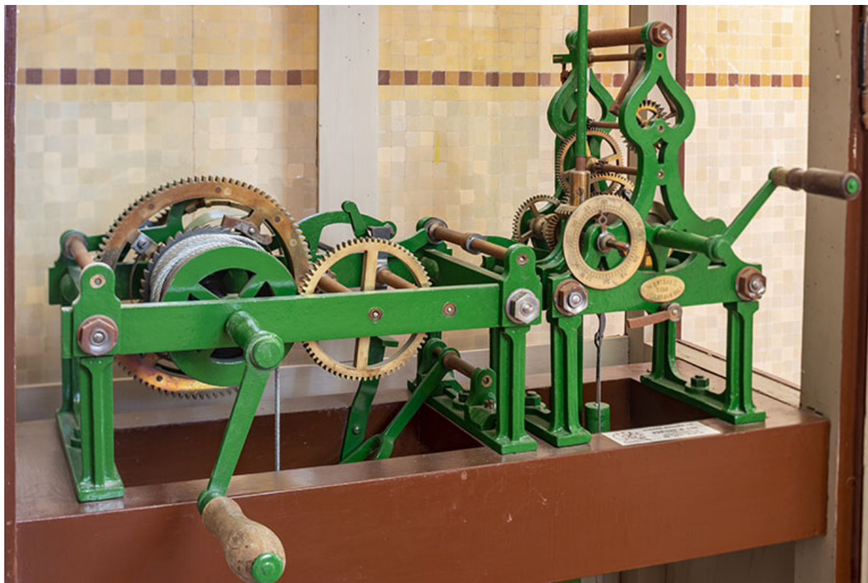
Vue du mécanisme avec ses manivelles.
