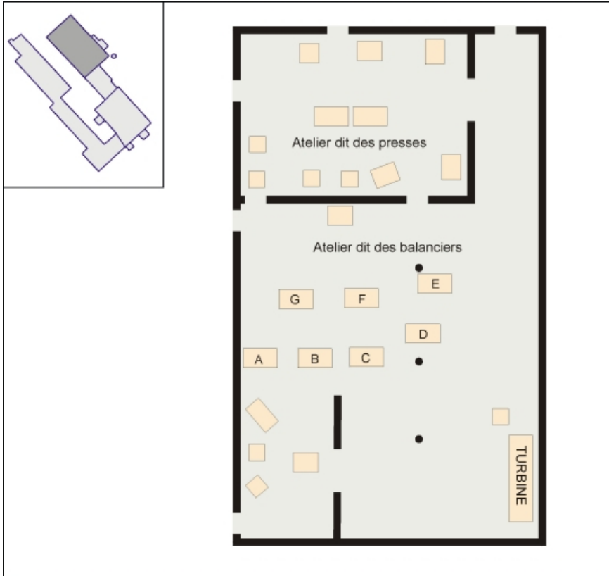
Plan de localisation des machines à estamper (presses à friction).
