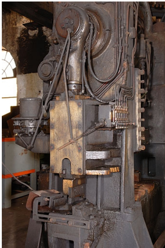
Détail des graisseurs et de la cisaille.
