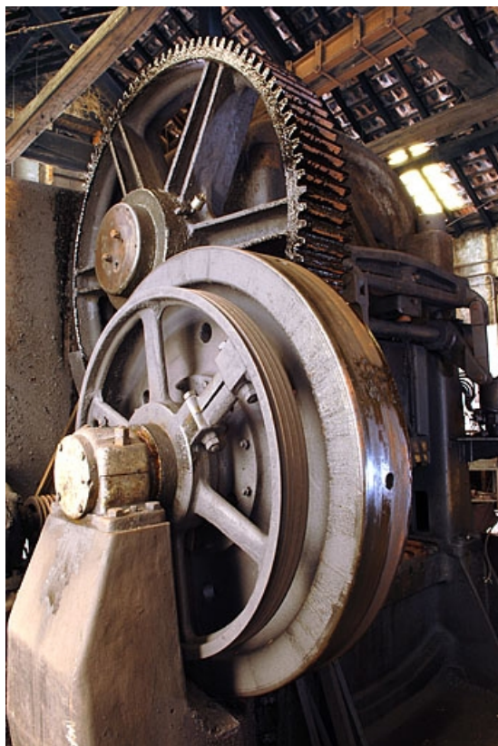
Détail des volants de transmission.
