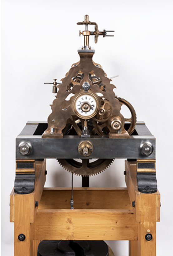
Mouvement : face avant.
