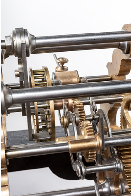
Mouvement : détail de l'échappement.
