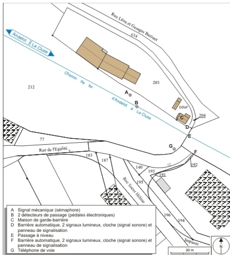
Plan de situation. Extrait du plan cadastral informatisé, 2006, section AE, échelle 1:1000. 39, Champagnole rue Léon et Georges Bazinet
