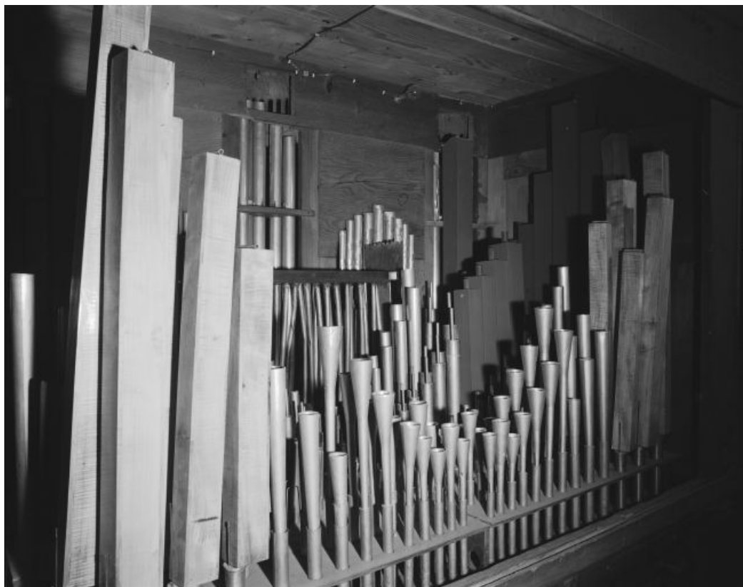
Tuyaute du clavier manuel, vu de trois quarts gauche.
