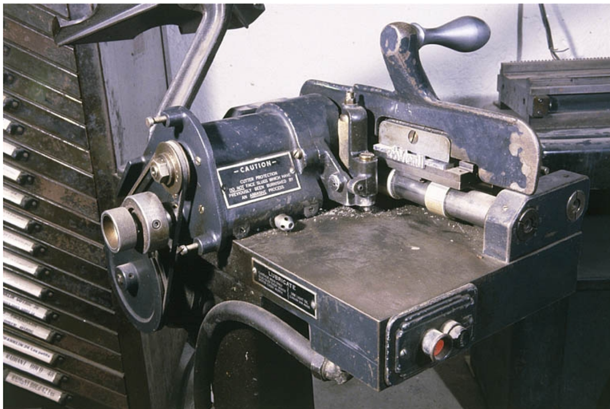
Détail : systèmes d'entraînement de la fraise et de fixation de la ligne-bloc. Une ligne-bloc est serrée dans la mâchoire. 39, Saint-Claude, 12 rue de la Poyat
