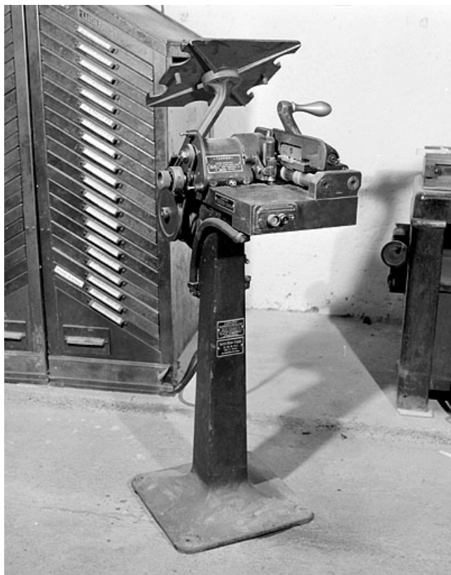
Vue d'ensemble d'une machine. Le support des lignes-blocs ("lutrin") est monté à l'envers (inclinaison vers l'arrière et non vers l'avant).
