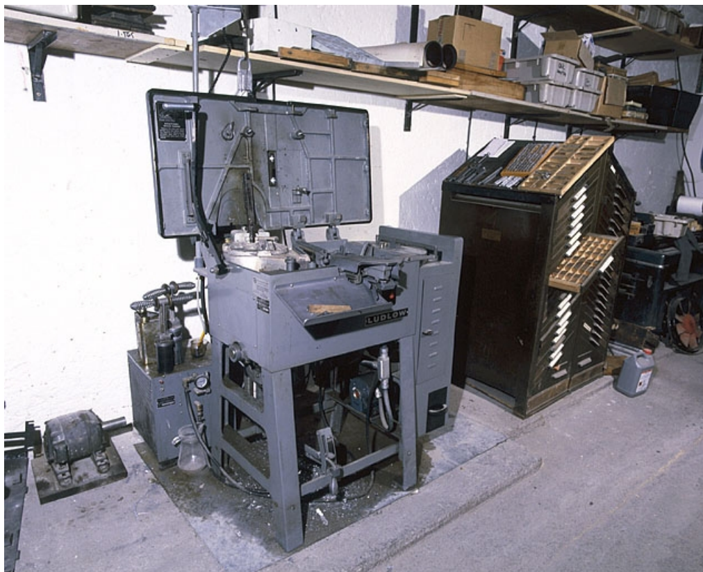
Fondeuse de lignes-blocs et 2 rangs à pupitre.
