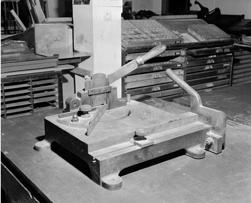
Vue d'ensemble d'un coupoir-biseautier. "Couteau-rabot" pour les coupes obliques à gauche, "couteau-guillotine" pour les coupes de longueur à droite.
