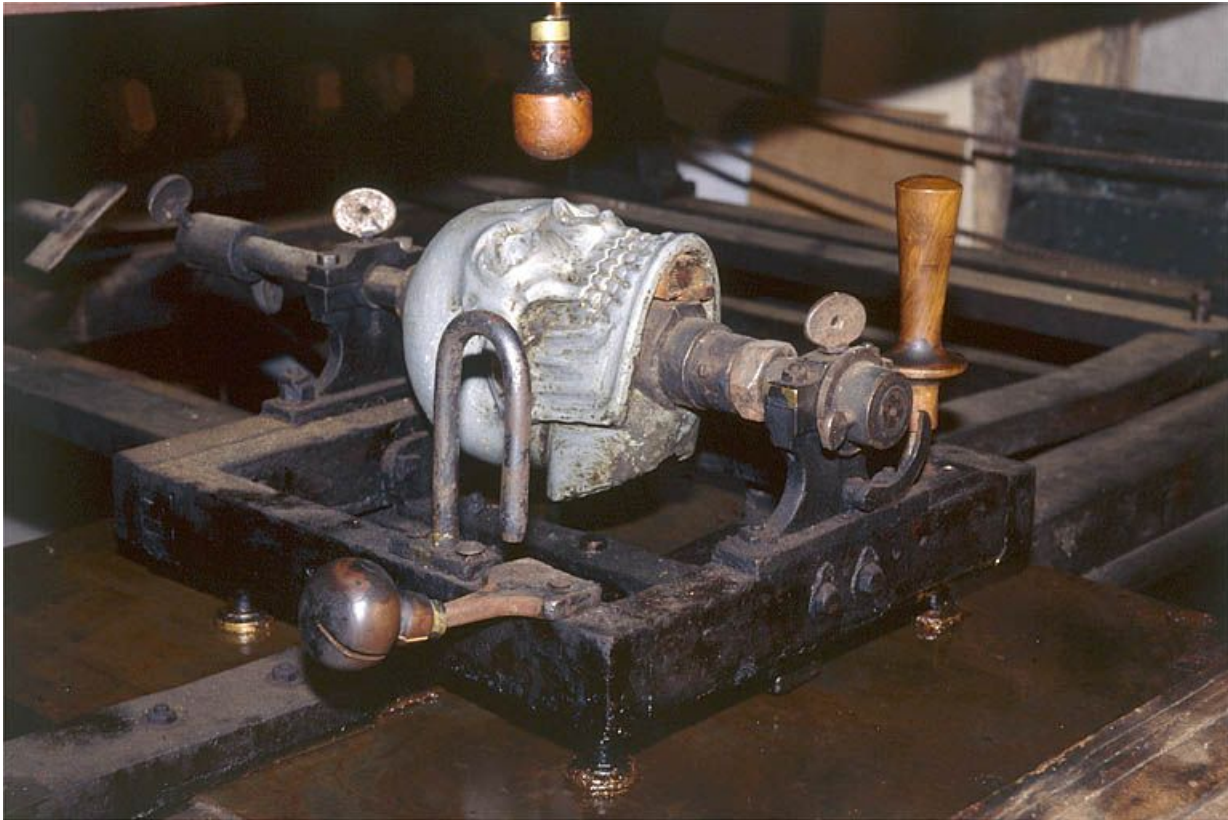
Support du modèle. Bougée à l'aide d'une poignée verticale et d'une poignée horizontale, cette partie du bâti mobile glisse sur une plaque métallique. Noter au-dessus du crâne l'extrémité du palpeur, laissé en position haute.
