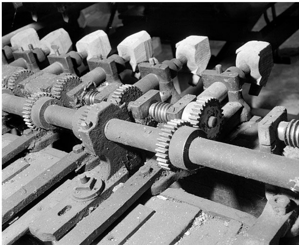
Face arrière : engrenages permettant la rotation simultanée des ébauchons.
