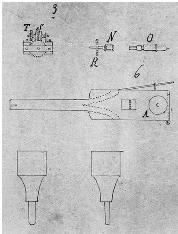
Dessins de détails [partie gauche du plan] : engrenages, système de rotation des supports d'ébauchons, fraises.
