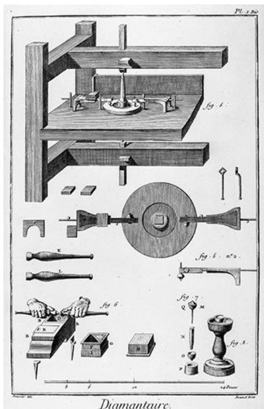
Diamantaire [banc de taille, pince (tenaille de lapidaire) et coquille (dop), débrutage ("égrisage")].
