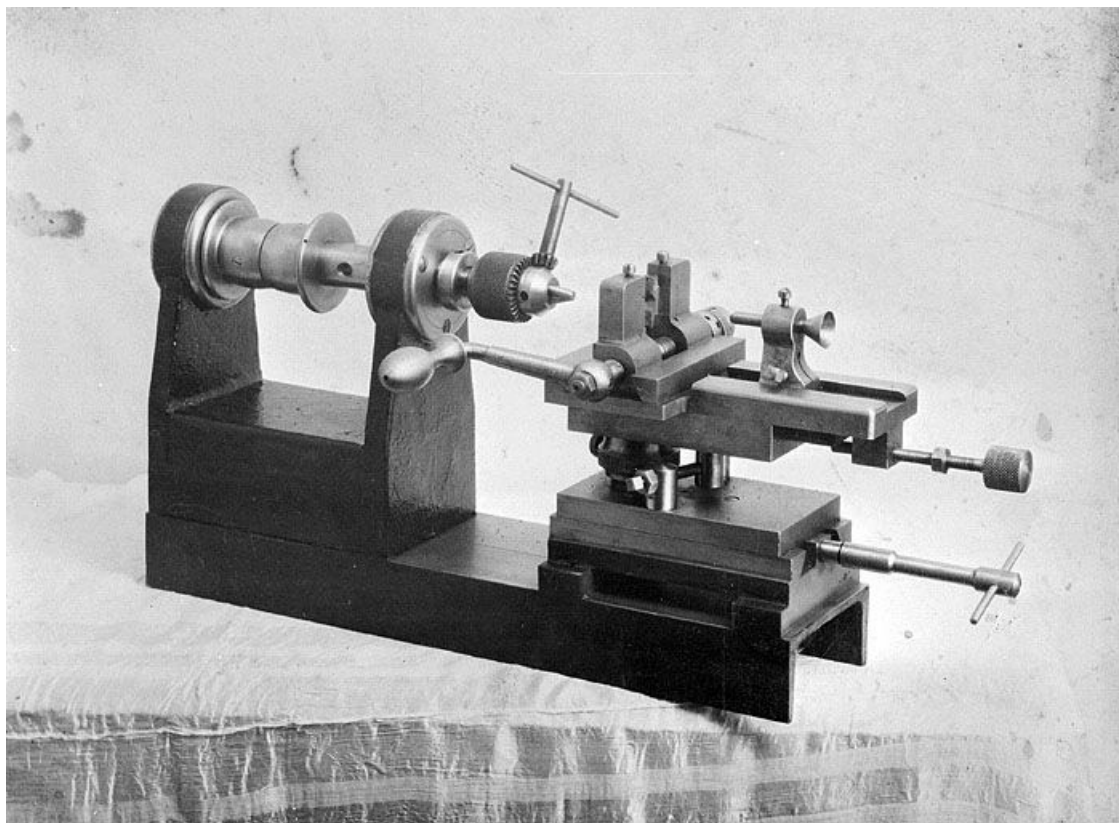
Exemple de machine à percer du constructeur mécanicien Lizon.
