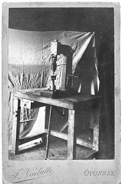
Exemple de machine à marquer du constructeur mécanicien Lizon.
