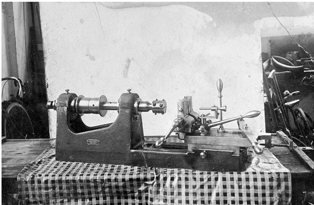
Exemple de machine à floquer du constructeur mécanicien Lizon.
