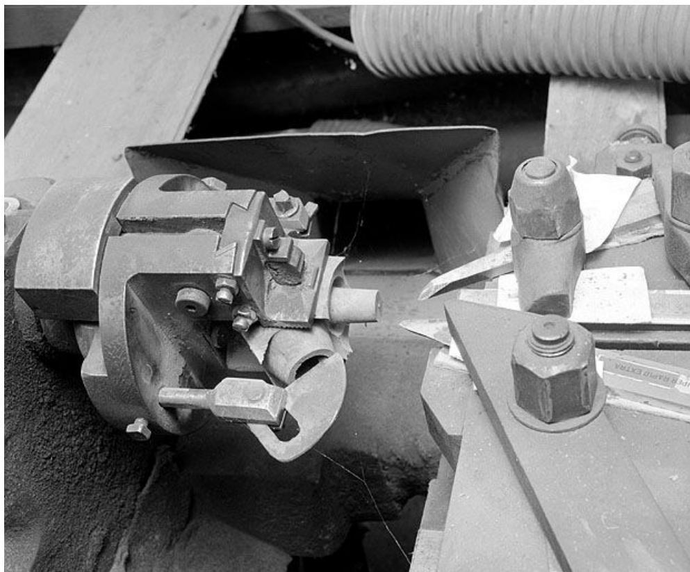
Vue rapprochée du mandrin gueule de loup et des outils.
