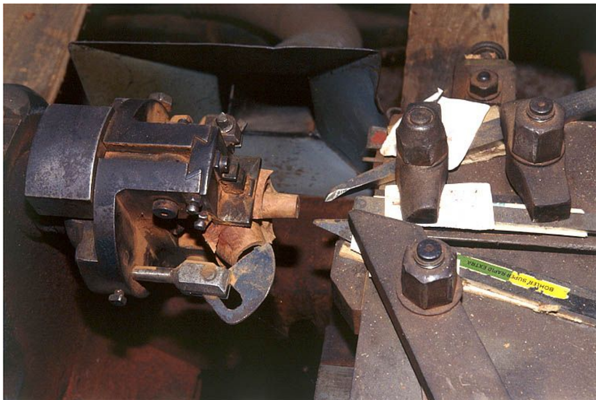
Vue rapprochée du mandrin gueule de loup et des outils.
