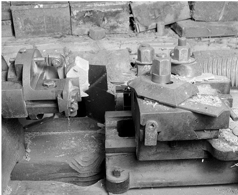
Mandrin gueule de loup et chariot porte-outils.
