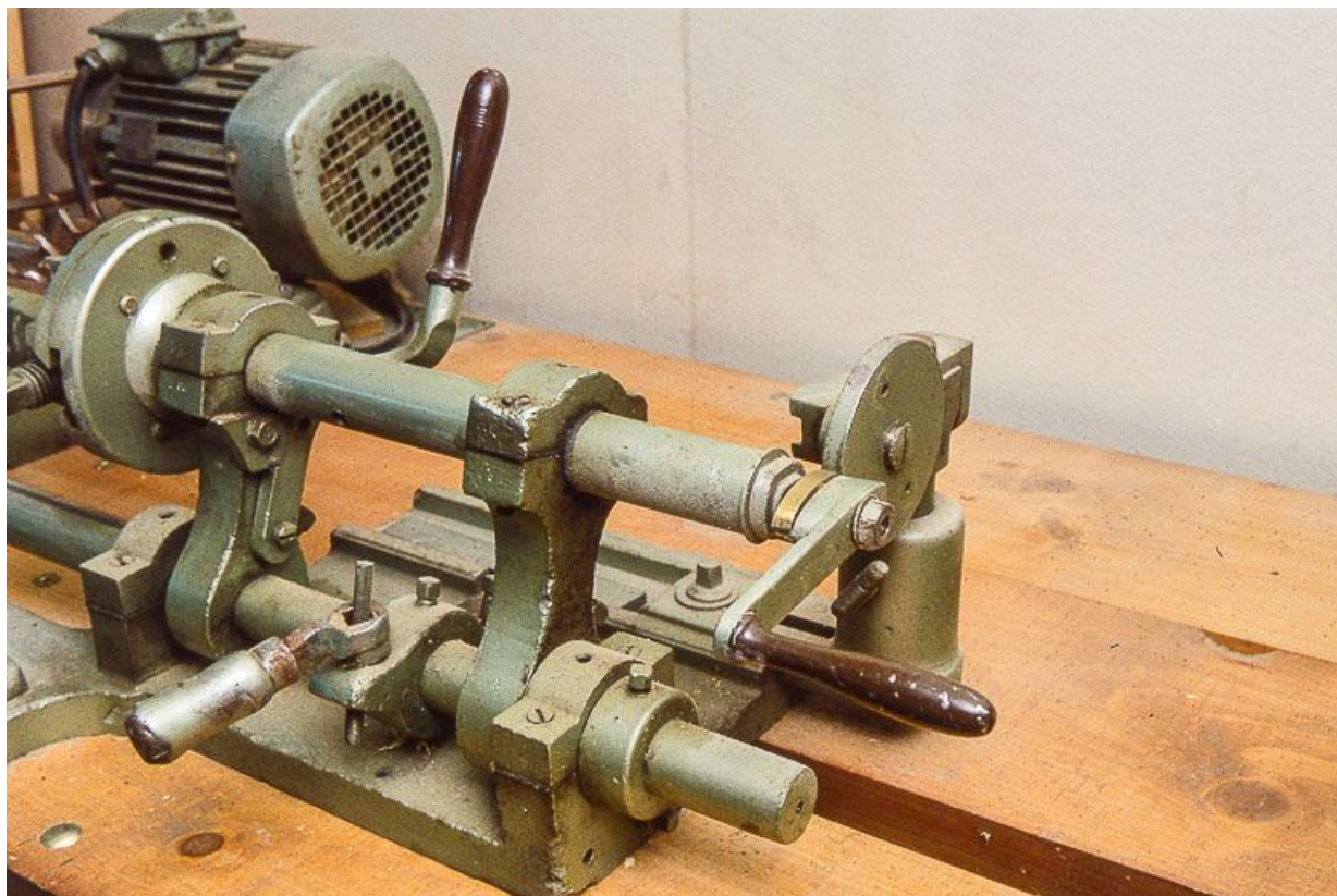
Détail du support de pièce : la came frottant contre la roue donne la forme et les cotes de la boîte de la tabatière.
