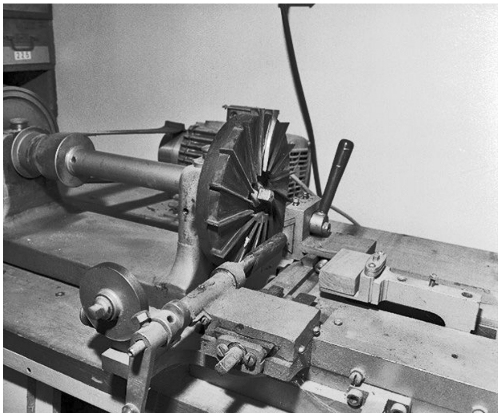
Détail du chariot et de la fraise.
