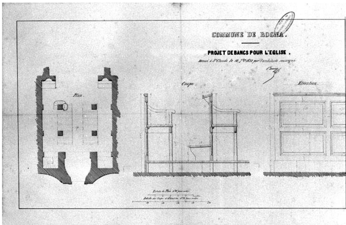
Commune de Rogna. Projet de bancs pour l'église [plan, coupe, élévation].
