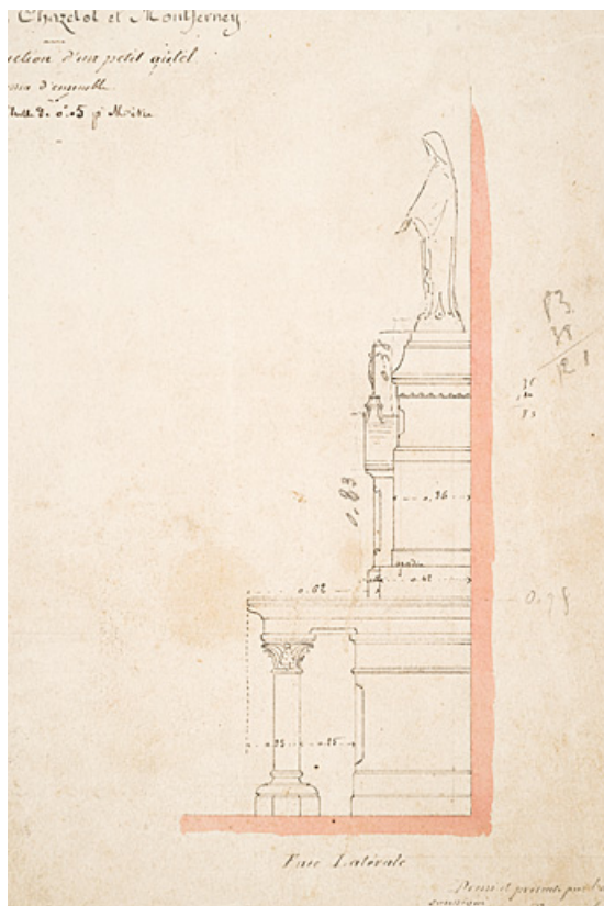
Communes de Chazelot et Montferney. Construction d'un petit autel. Dessin d'ensemble. [Détail :] Face latérale. 23 mars 1872. 25, Rougemont, lieudit : Saint-Hilaire
