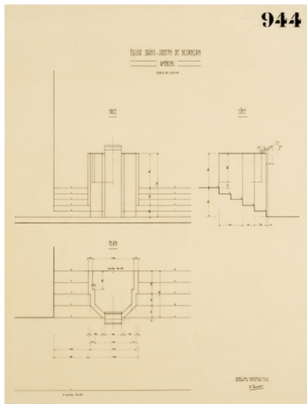
Plan et élévations des ambons de l'église Saint-Joseph. Juillet 1954. 25, Besançon, 18 avenue Villarceau
