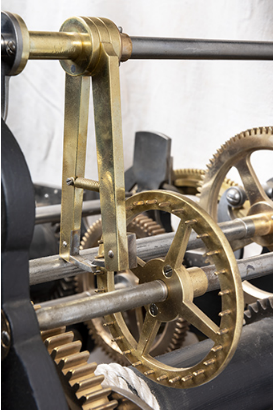
Mouvement, mécanisme des heures : échappement à chevilles.
