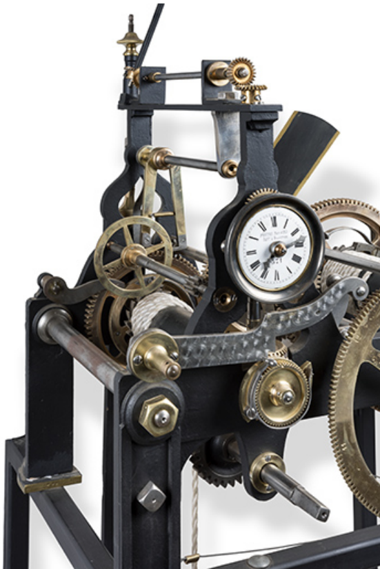
Mouvement : mécanisme des heures.
