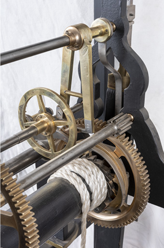
Mouvement, mécanisme des heures : échappement à chevilles et tambour moteur. 25, Mamirolle, 10 rue des Quatre Vents
