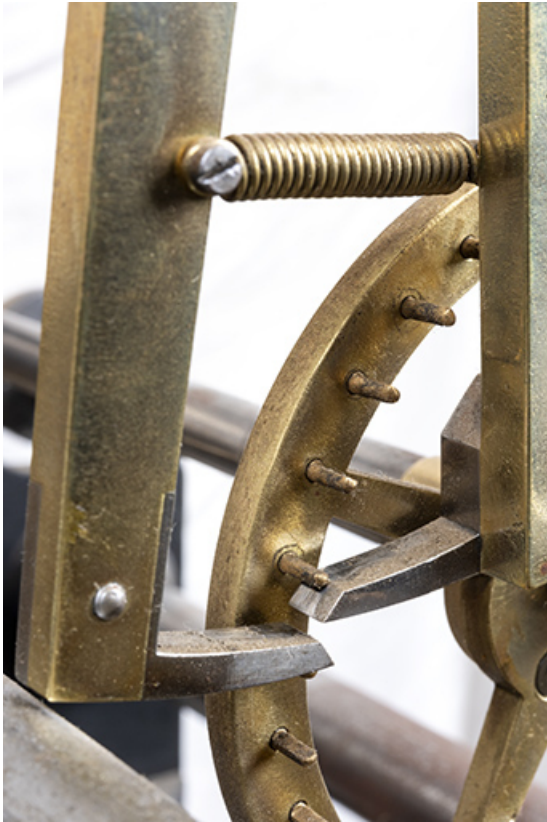
Mouvement, mécanisme des heures : échappement à chevilles (détail de l'ancre et des chevilles). 25, Mamirolle, 10 rue des Quatre Vents
