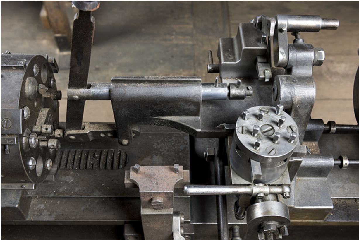
Vue plongeante sur la partie travaillante. Tourelle revolver au premier plan.
