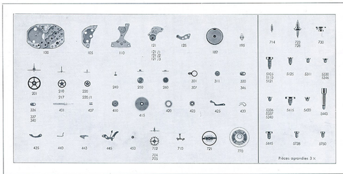
Calibre 5 1/4''' - 55 - 15 à 21 rubis [éclaté des fournitures], 1973.
