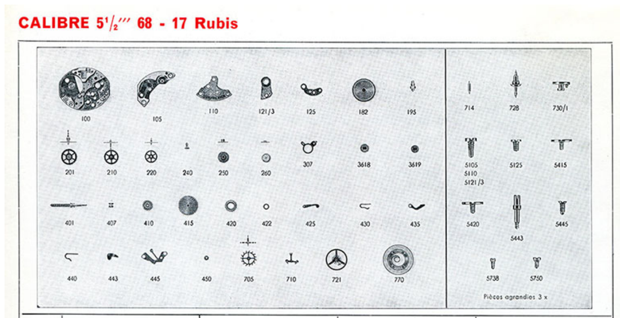
Calibre 5 1/2''' 68 - 17 rubis [éclaté des fournitures], 1973. 25, Maîche
