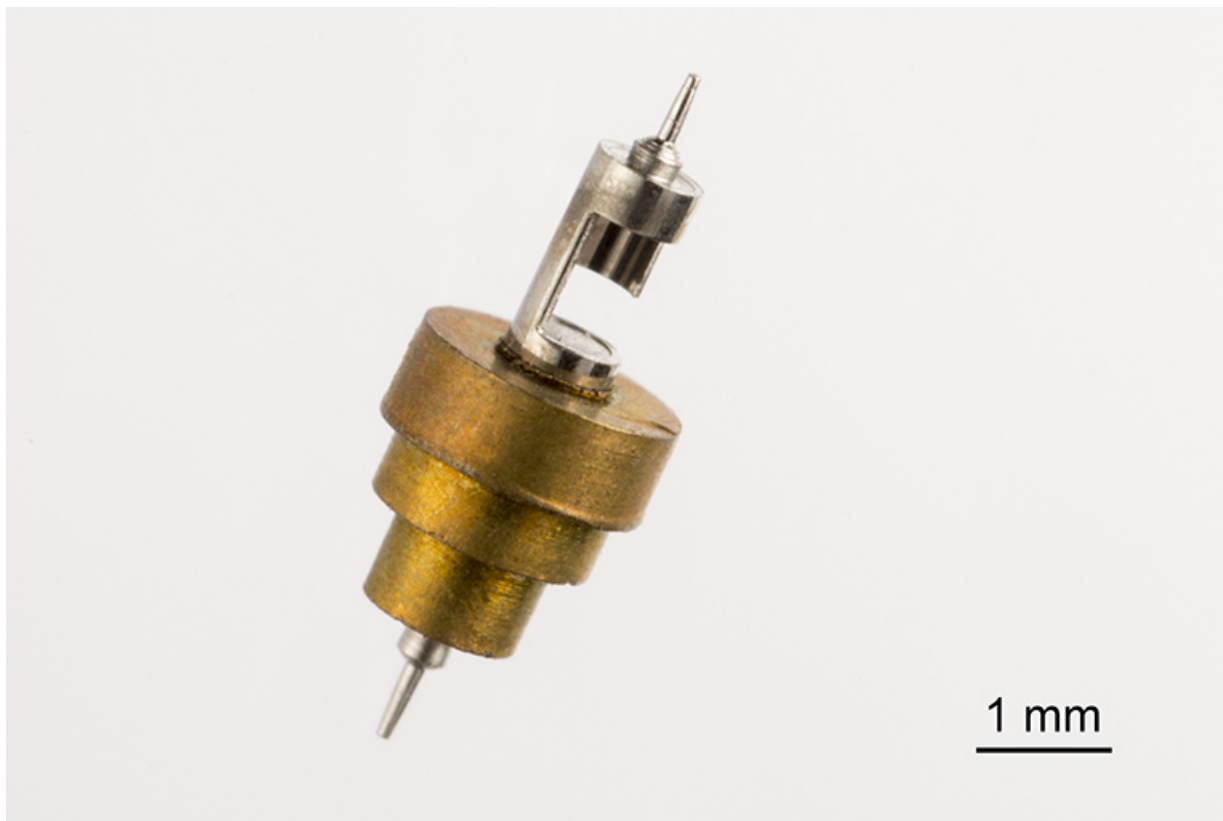
Echappement à cylindre : cylindre (en métal blanc) équipé de la "siette" (assise du balancier) en laiton. 25, Charquemont, 12 Rue Neuve
