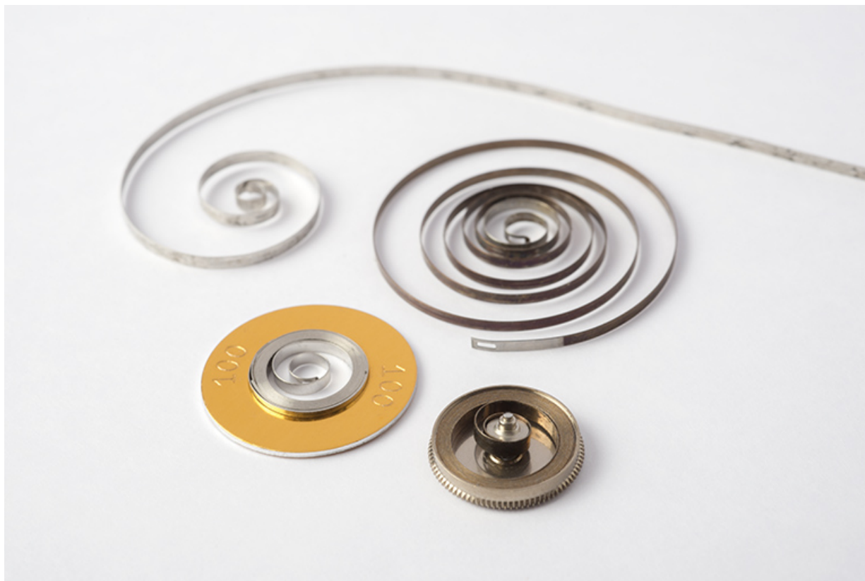
Barillet démonté et ressorts moteurs. Un ressort est visible dans la boîte du barillet.
