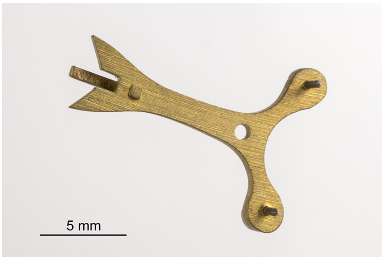
Echappement à chevilles : ancre (les chevilles sont visibles à droite).
