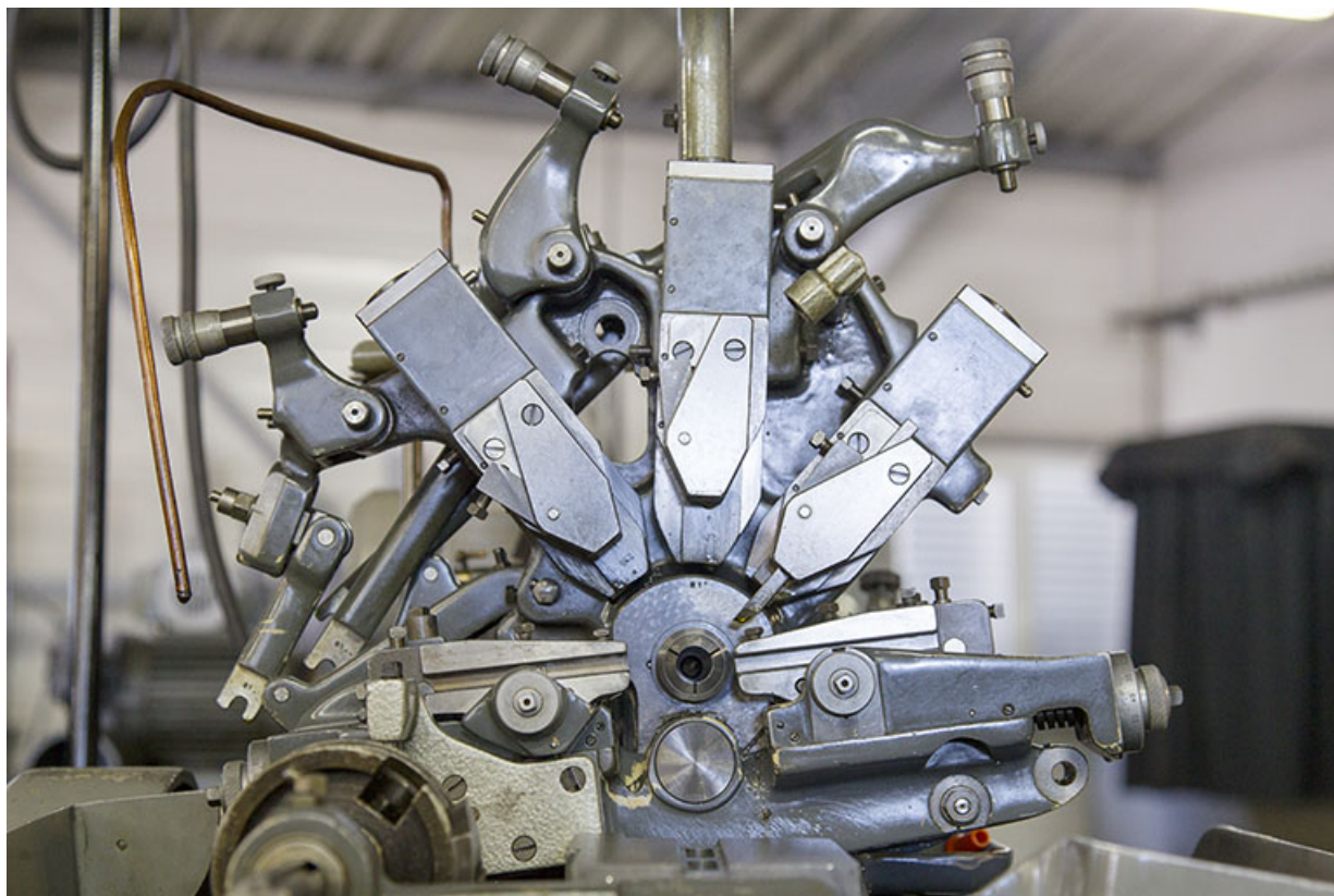
La lunette à bascule, avec ses cinq porte-burins.
