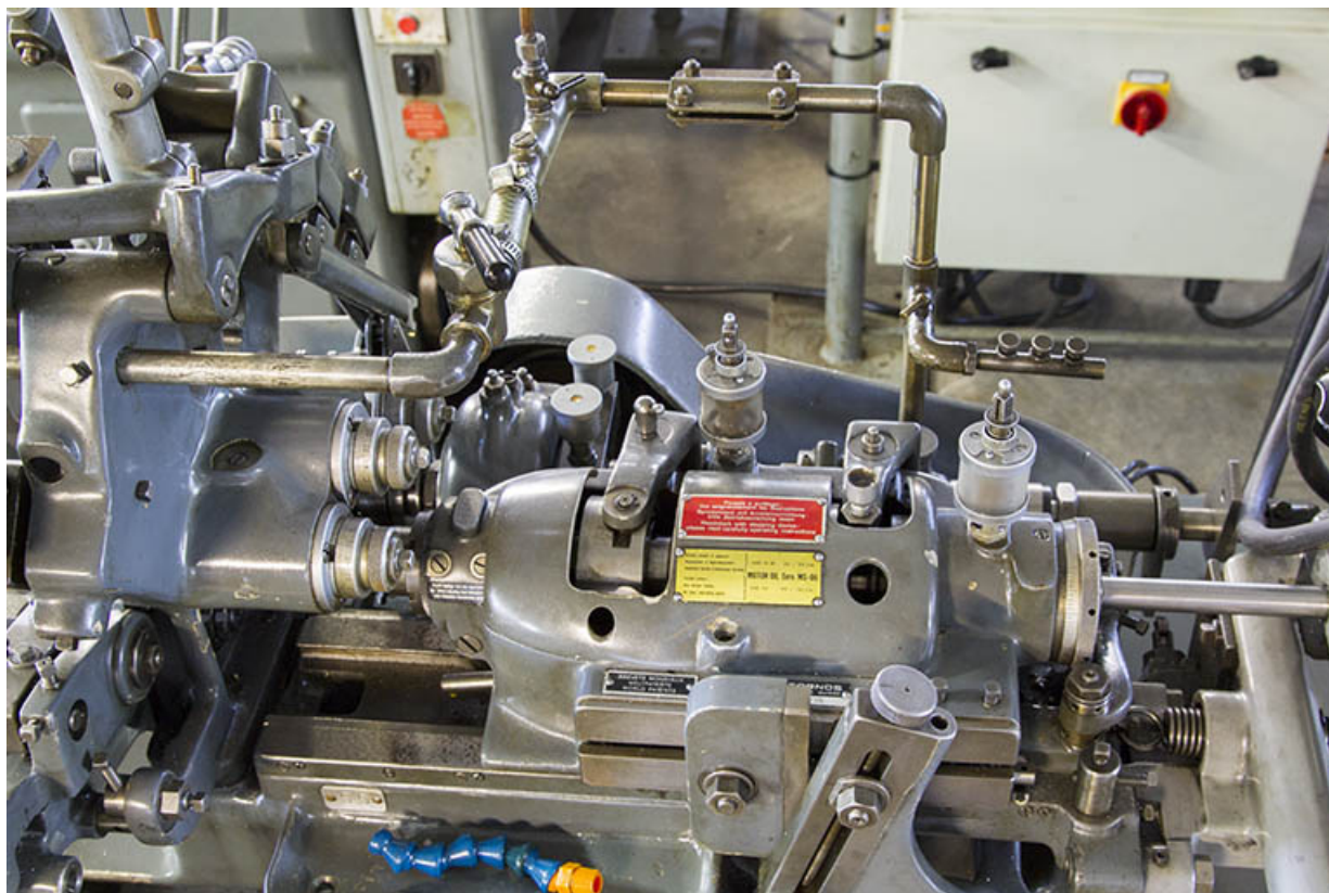
Vue plongeante sur la poupée mobile et le système de lubrification.
