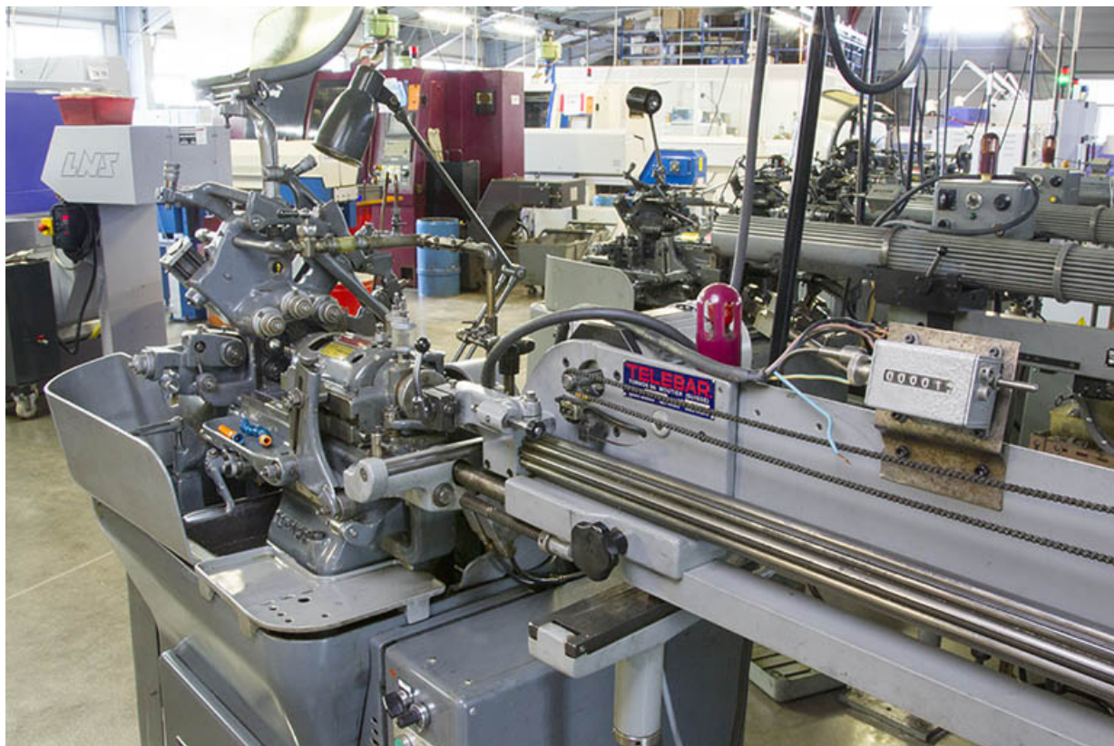
La machine côté poupée mobile et son ravitailleur.
