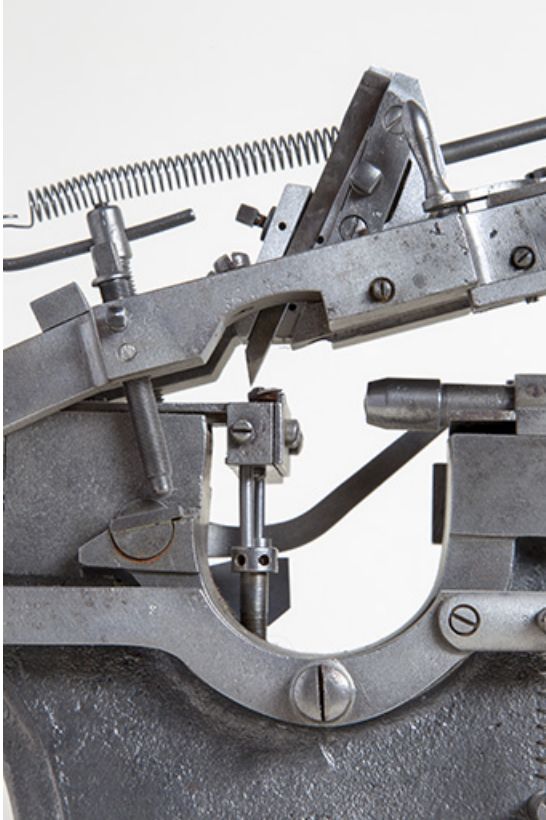
Espace d'usinage : burin en haut, tube guide-fil à droite.
