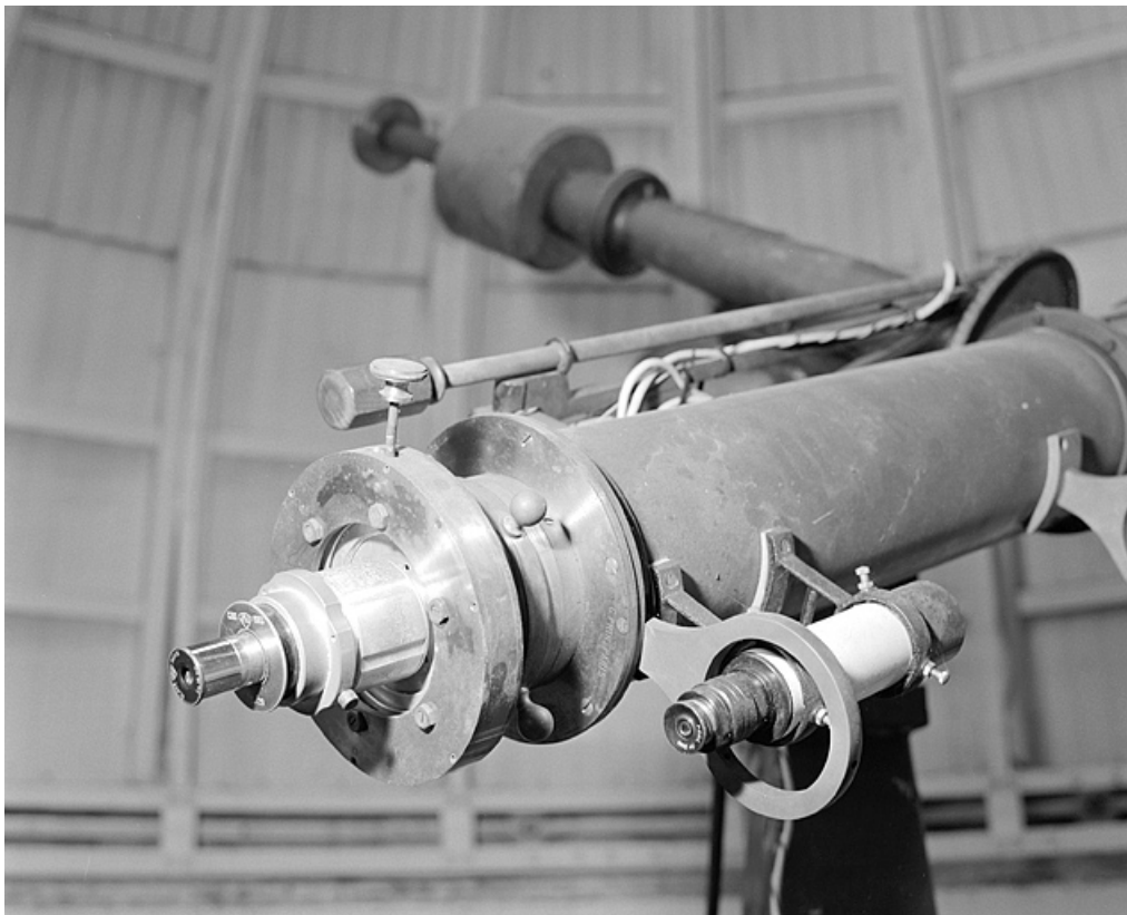
Partie oculaire de la lunette équatoriale Prin.
