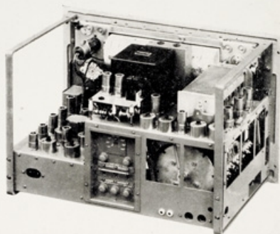
Le chassis du 2 e changeur de fréquence, est représenté non muni de son capot de blindage.
