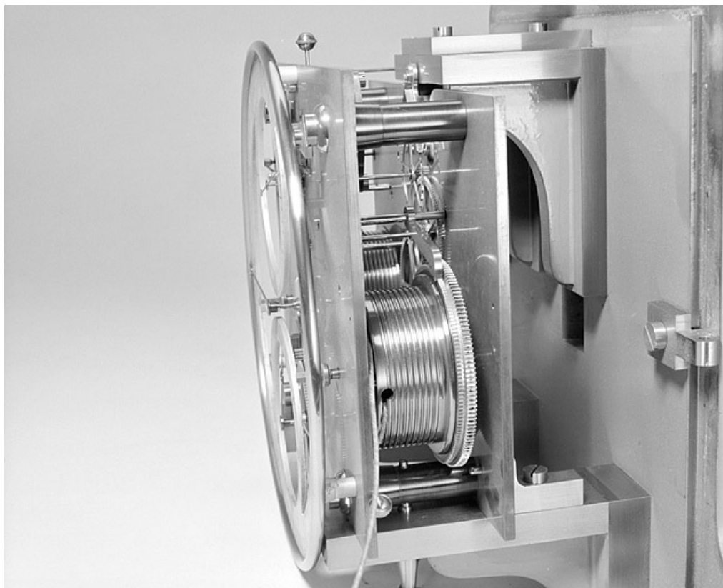
Vue latérale montrant le mouvement à deux corps de rouages, monté entre deux platines en laiton.
