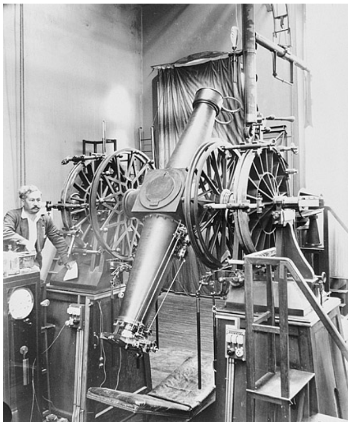
[Vue d'ensemble de la lunette méridienne], limite 19e siècle 20e siècle.
