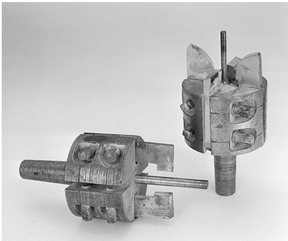
Détail de deux outils de coupe.
