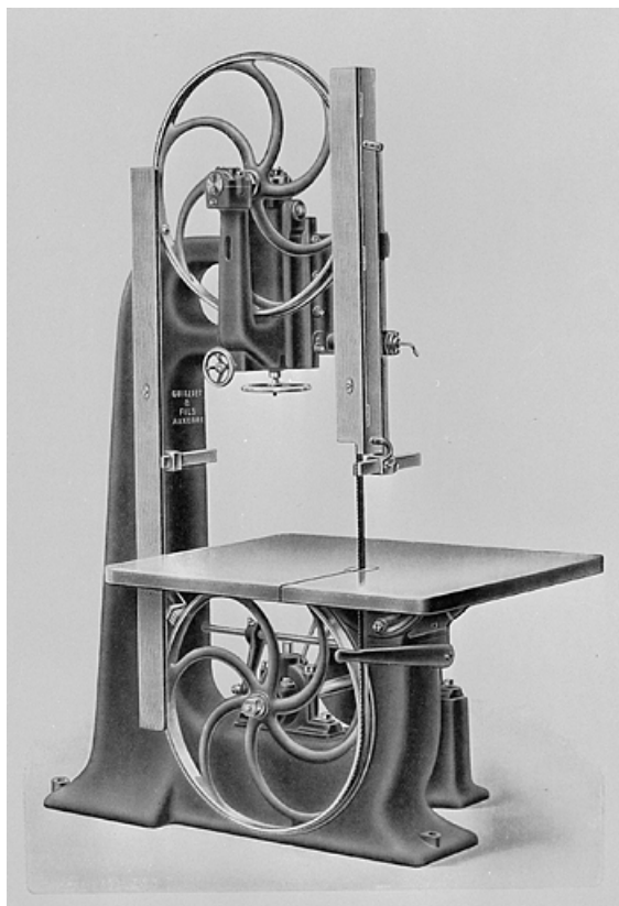
Scie à ruban à table inclinable.
