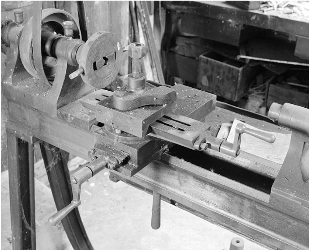
Le trainard entre la poupée fixe et la poupée mobile.
