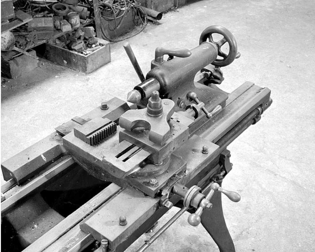
Détail du trainard et de la poupée mobile.
