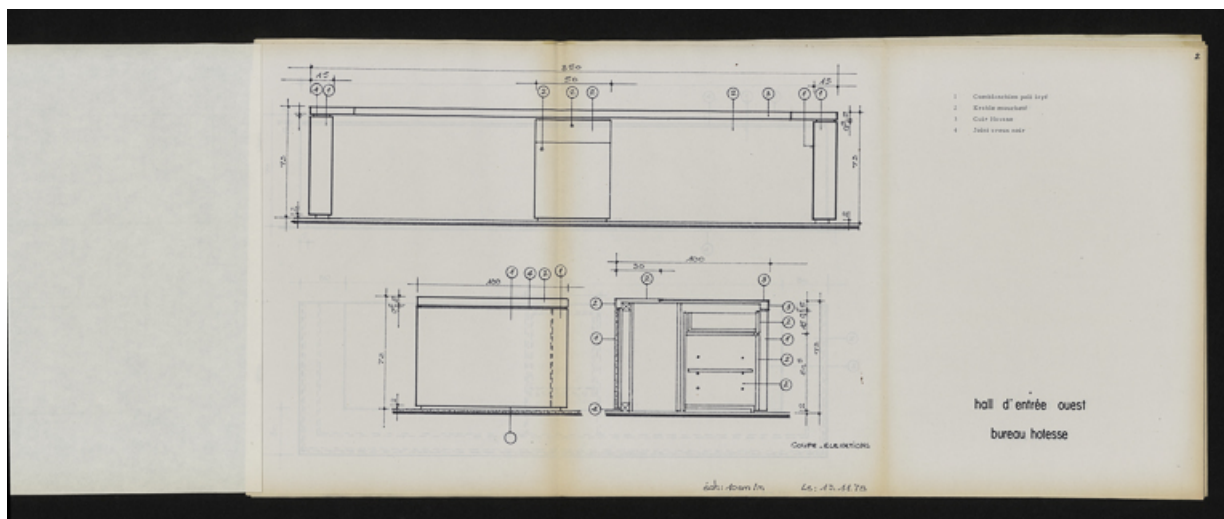
Carnet de détails et principes - hall d'entrée ouest : bureau des hôteses, coupe et élévations, 13 novembre 1978. Boyer, Michel (architecte d'intérieur) (Archives départementales de la Côte-d'Or, Dijon, 32 J 106)
