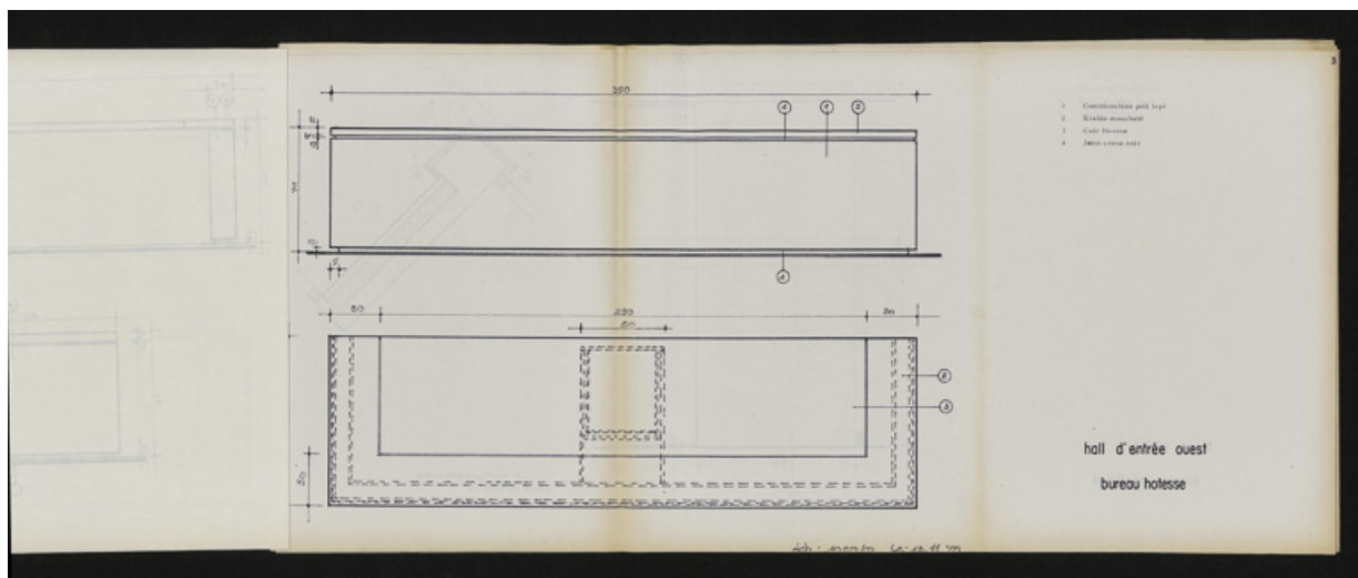
Carnet de détails et principes - hall d'entrée ouest : bureau des hôtes, plan et élévation, 13 novembre 1978. Boyer, Michel (architecte d'intérieur) (Archives départementales de la Côte-d'Or, Dijon, 32 J 106)
