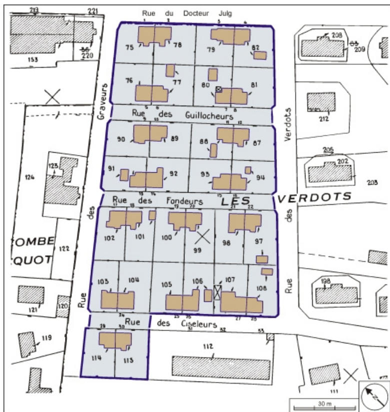
Plan-masse et de situation. Extrait du plan cadastral, 1979, section AC, 1:1000. 90, Beaucourt, lieudit : cité Adolphe Japy
