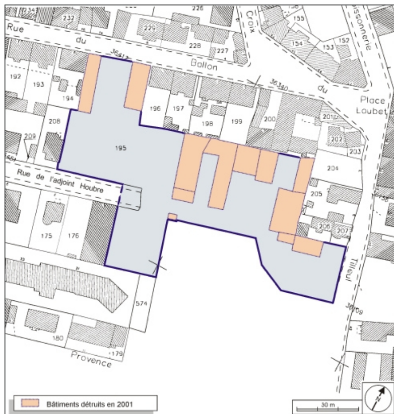
Plan-masse et de situation. Extrait du plan cadastral, 2001, section AH, 1:1000. 90, Belfort rue de l' Adjoint Houbre
