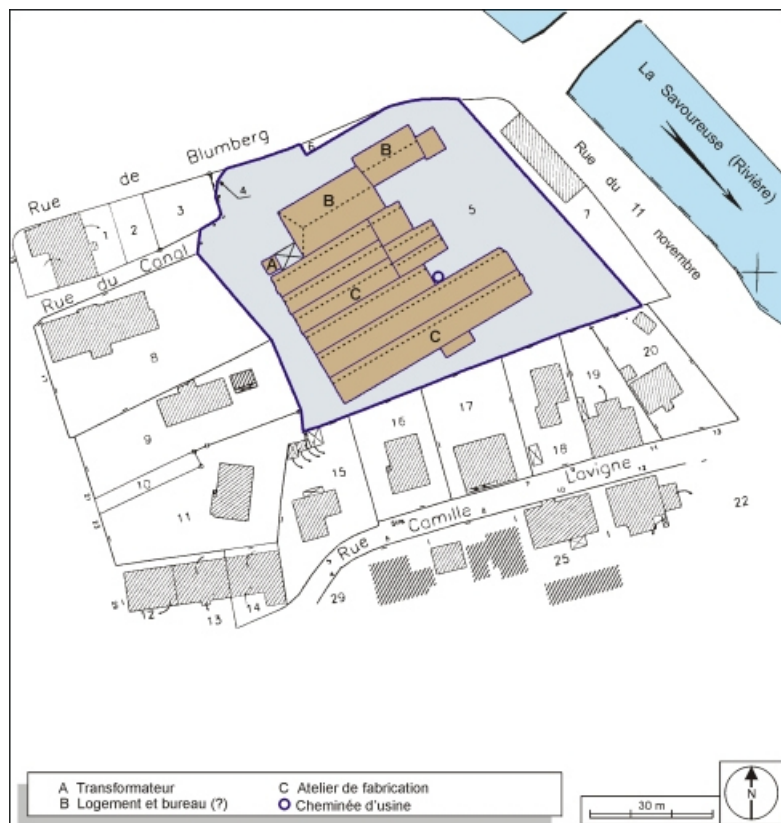
Plan-masse et de situation. Extrait du plan cadastral, 2000, section BI, 1:1000. 90, Valdoie rue de Blumberg
