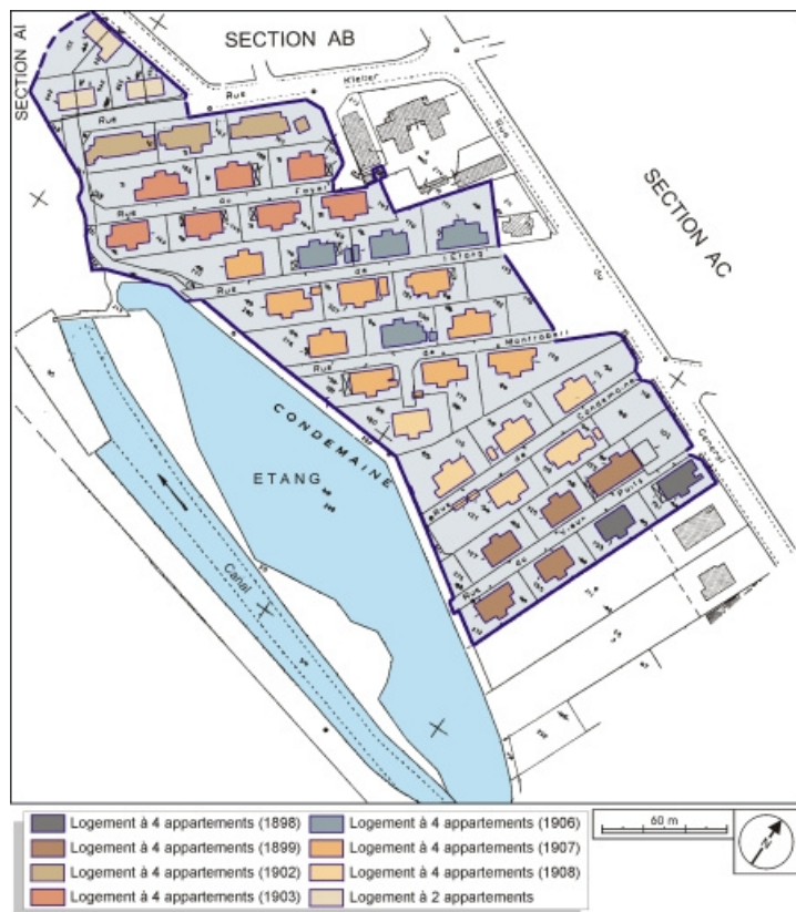
Plan-masse et de situation. Montage d'extraits de plan cadastral, 1984, sections AH et AI, 1:000, le tout réduit à 1:2000. 90, Grandvillars, lieudit : cité Condemaine
