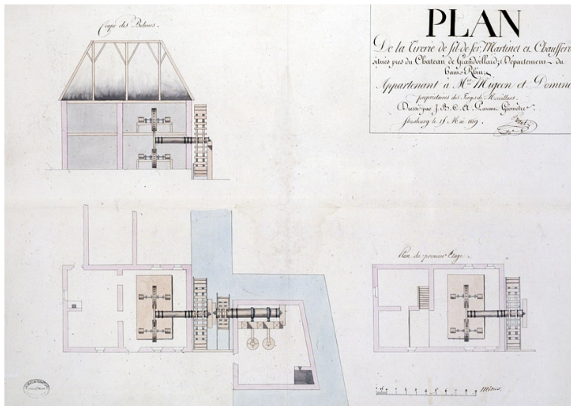
Plan de la tirerie de fil-de-fer, martinets et chaufferie, situés près du Château de Grandvillars [coupe transversale, plan au sol et plan du 1er étage].
