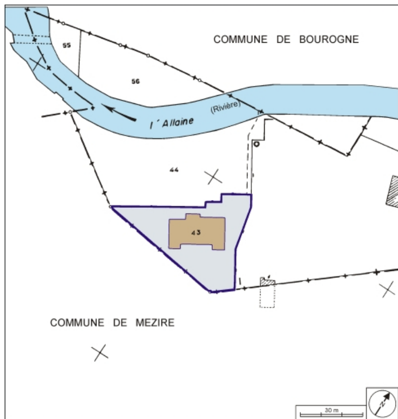
Plan-masse et de situation. Extrait du plan cadastral, 1984, section C, 1:1000. 90, Morvillars rue du Canal
