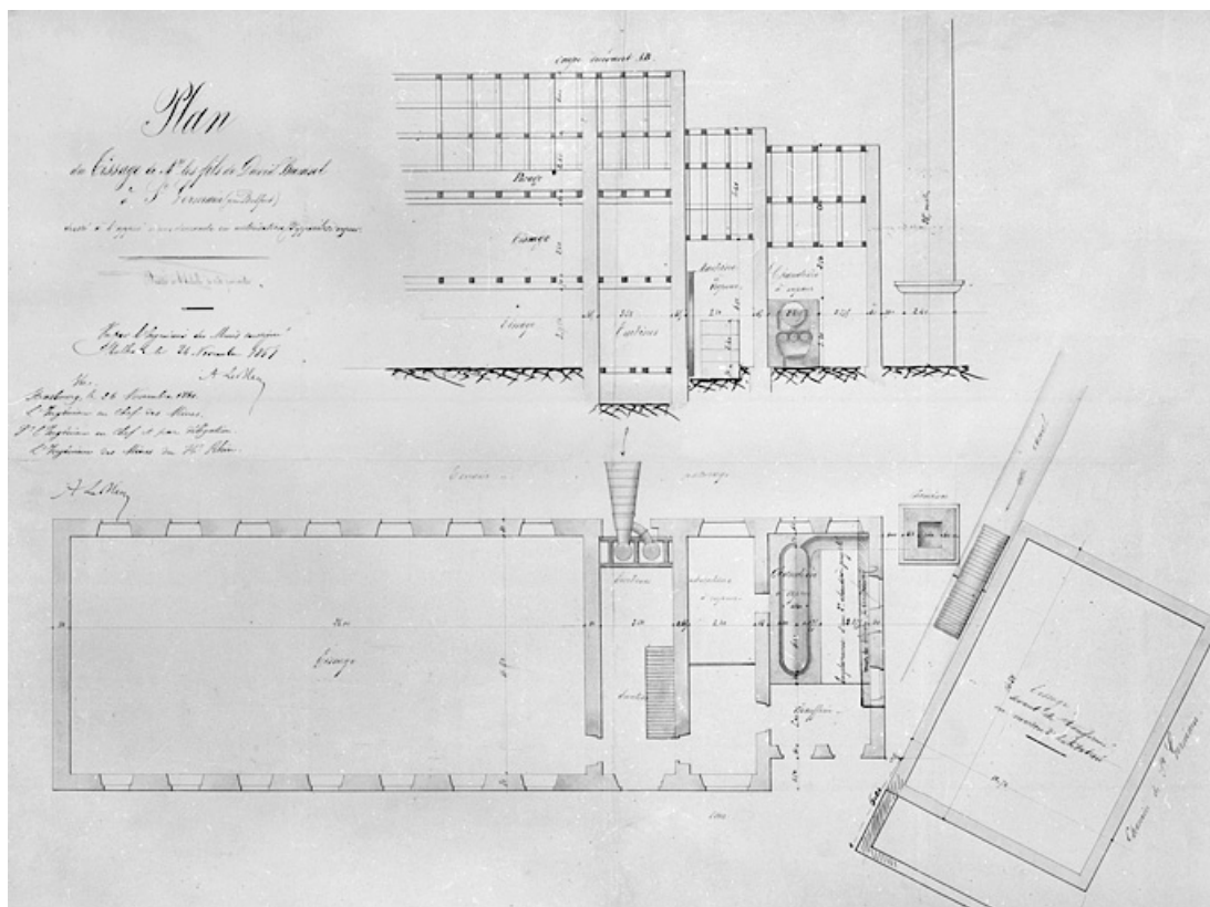
Plan du tissage de Mrs les fils de David Bumsel à Saint-Germain (près Belfort) dressé à l'appui d'une demande en autorisation d'appareils à vapeur.
