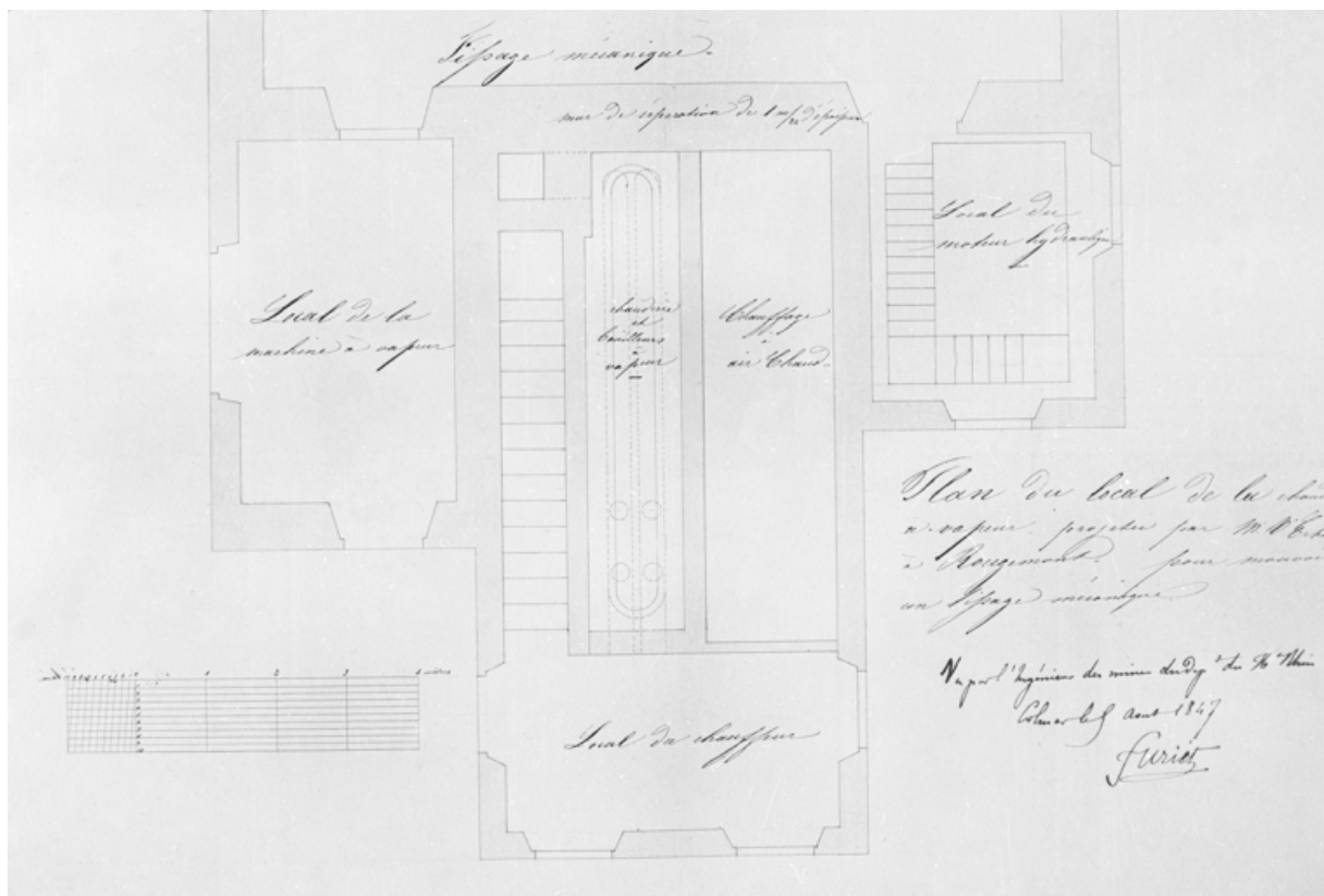
Plan du local de la chaudière à vapeur projetée par M. Erhard à Rougemont pour mouvoir un tissage mécanique. 90, Rougemont-le-Château, 24 rue Jean Moulin
