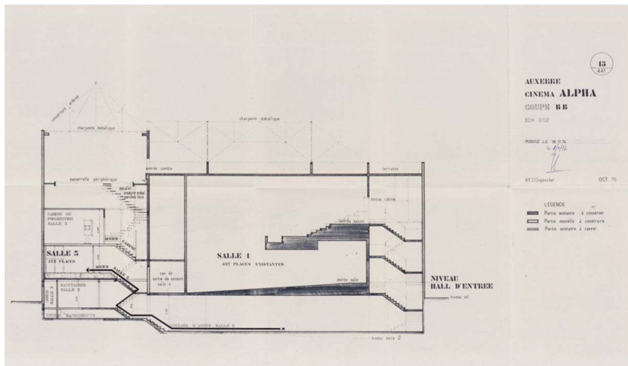
Auxerre. Cinéma Alpha. Coupe BB. 1976. 89, Auxerre
