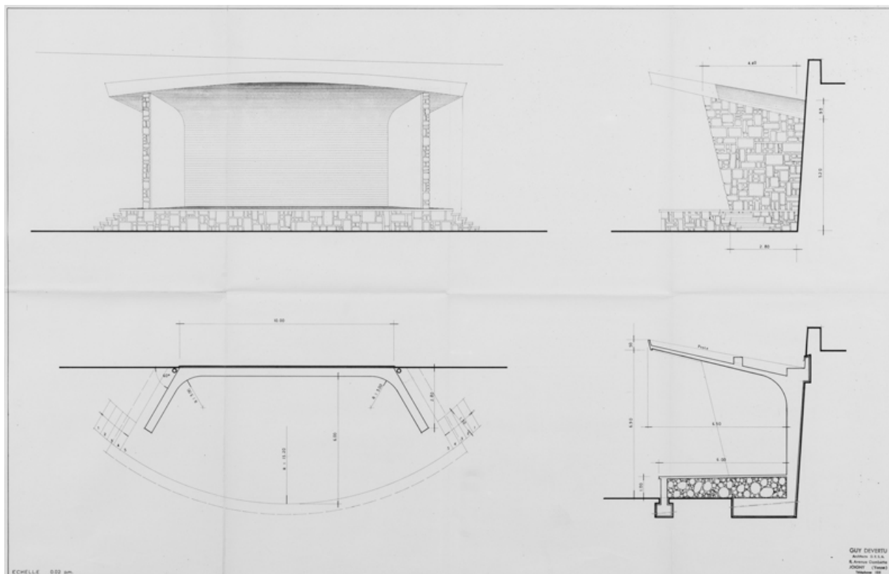
[Plan, coupes et élévation]. S.d. [1969].
