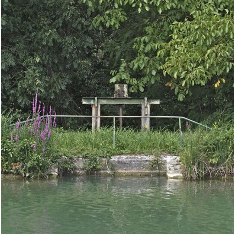
Le déversoir vu du canal : maçonnerie du déversoir, garde-corps et vanne.
