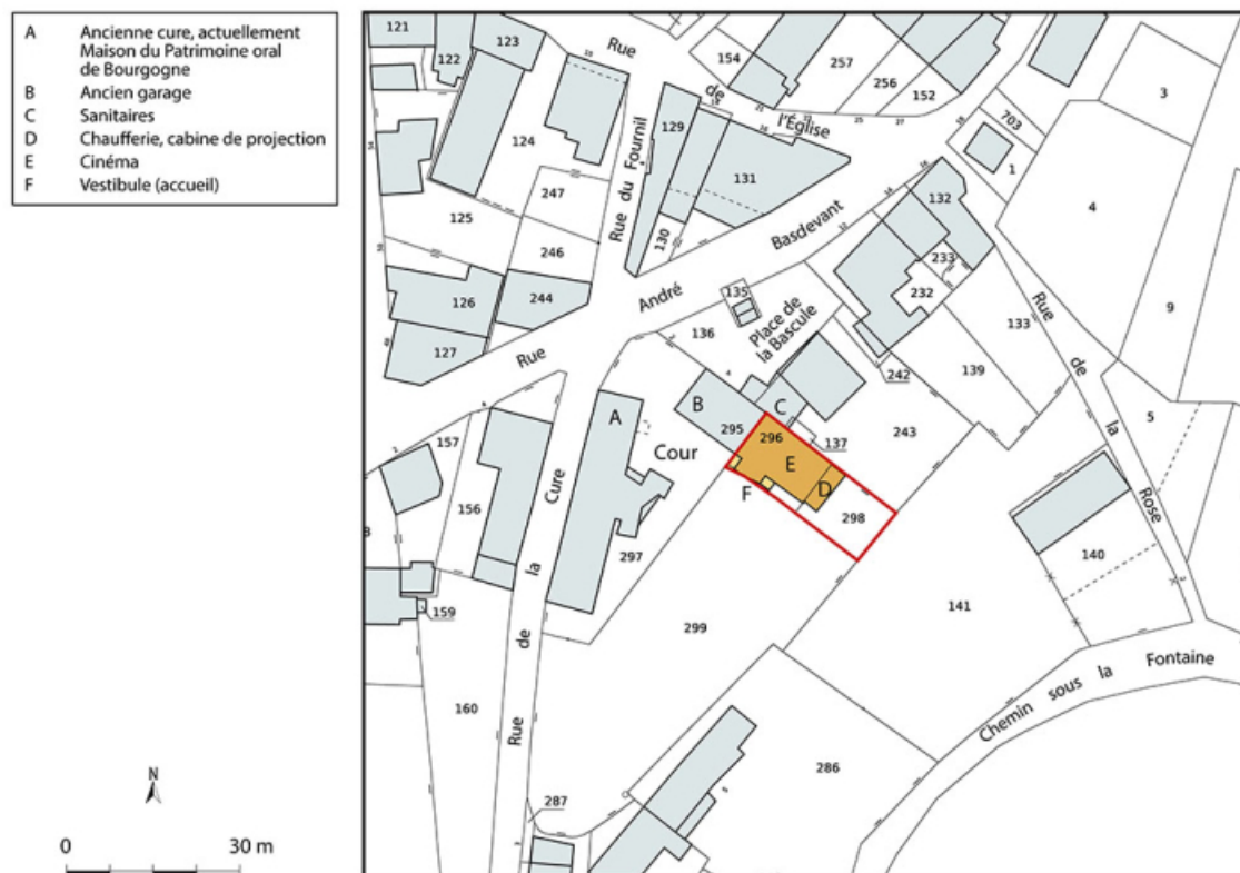
Plan-masse et de situation. Extrait du plan cadastral de la Direction Générale des Finances Publiques (DGFiP), 2022, section AE, 1/1 000 agrandi à 1/750.
