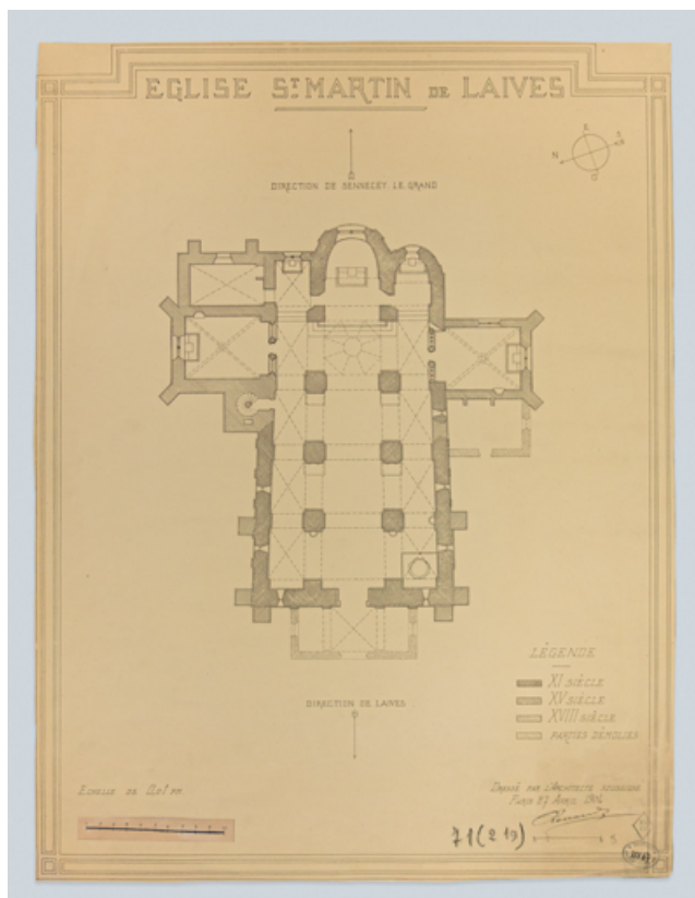
Plan de l'église relevé en 1904.
