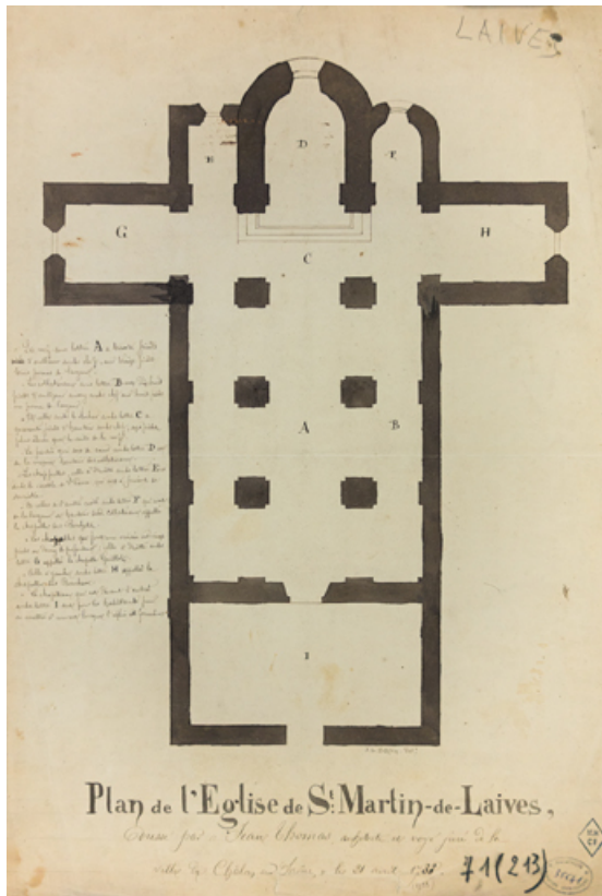
Plan de l'église relevé en 1733.
