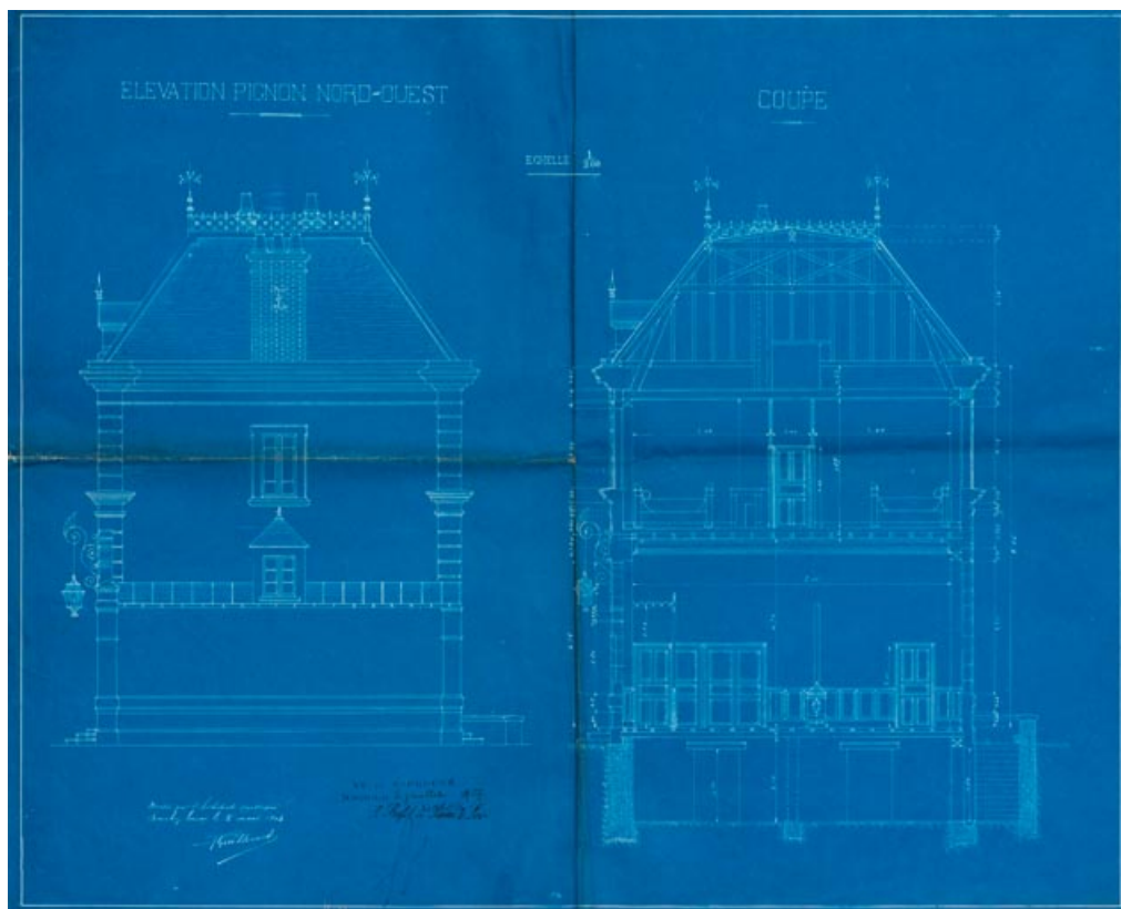
Élévation de la façade latérale et coupe. 71, Bourbon-Lancy place de la République
